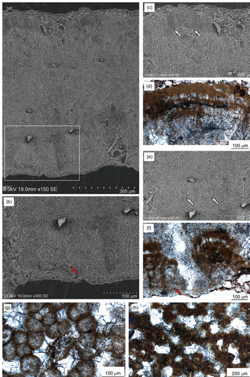
图 4 休宁伞形蛋(新蛋属, 新蛋种)蛋壳显微结构。(a) 蛋壳切面扫描电子显微镜(SEM)观察; (b) 单个半球形的锥体扫描电子显微镜观察((a)中方框部分)及其晶核中心(红色箭头所指); (c), (d) 柱状层近外表面处壳单元的伞形结构((c)为扫描电子显微镜(SEM)观察, (d)为组织学切片的普通光观察), 伞形结构由大块的方解石晶体组成((c)中白色箭头所指); (e), (f) 锥体层与柱状层过渡处壳单元的伞形结构((e)为扫描电子显微镜(SEM)观察, (f)为组织学切片的普通光观察), 伞形结构由大块的方解石晶体((e)中白色箭头所指), (f)中红色箭头所指为锥体的晶核中心; (g) 蛋壳锥体层弦切面, 示排列疏密不均的锥体, 锥体呈半球形沿晶核中心向外呈放射状生长, 部分锥体紧密相连; (h) 蛋壳柱状层中上部弦切面, 示间隔明显的壳单元和不规则气孔
